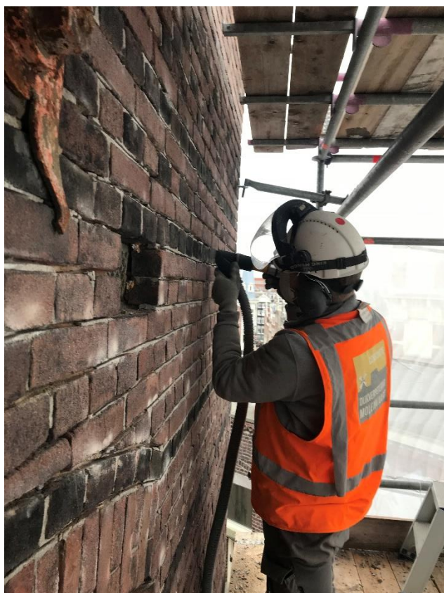
Figuur 3 Uitslijpen en uithakken van het bestaande voegwerk/metselwerk
