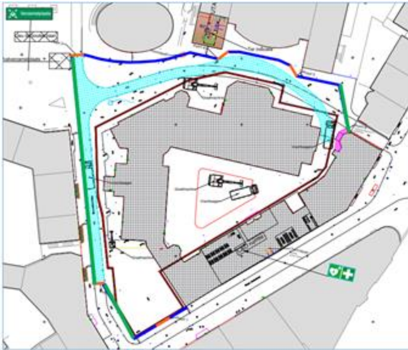
Figuur 1: Bouwterrein UB, kader om terrein markeert bouwhek.
